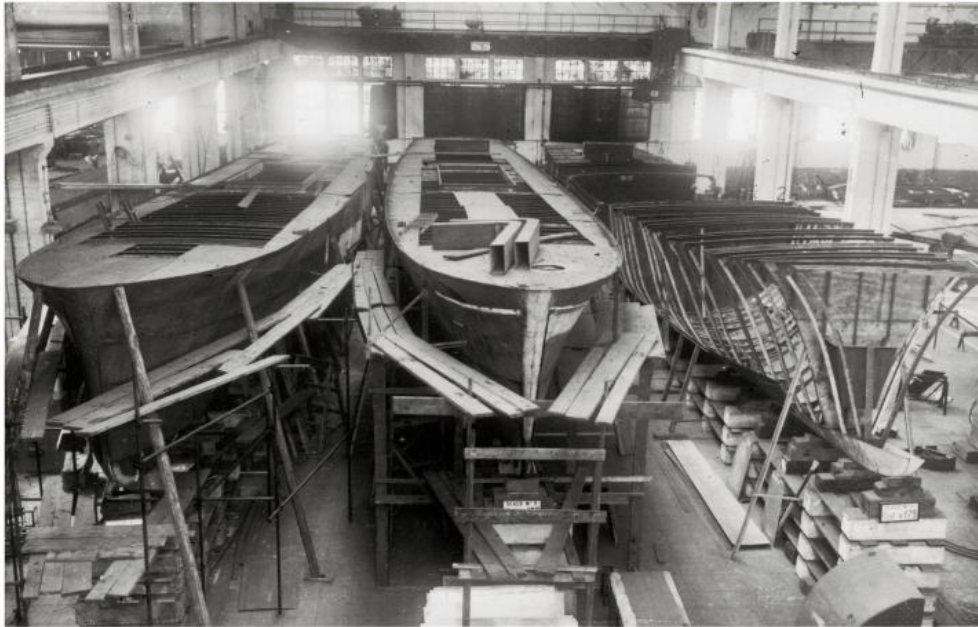
VAS 305 , VAS 306 E VAS 304 - 1942 CANTIERE CERUSA GENOVA VOLTRI
